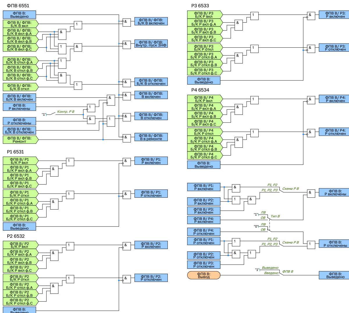
Рисунок 2.61 – Функциональная схема логики ФПВ В2
