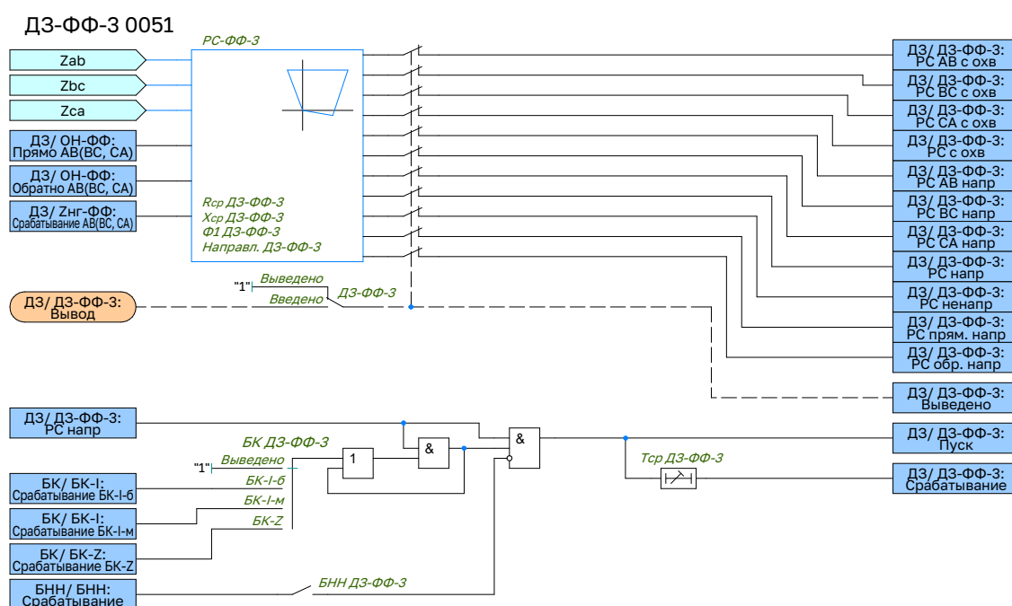
Рисунок 2.12 – Функциональная схема логики ДЗ-ΦΦ-3
