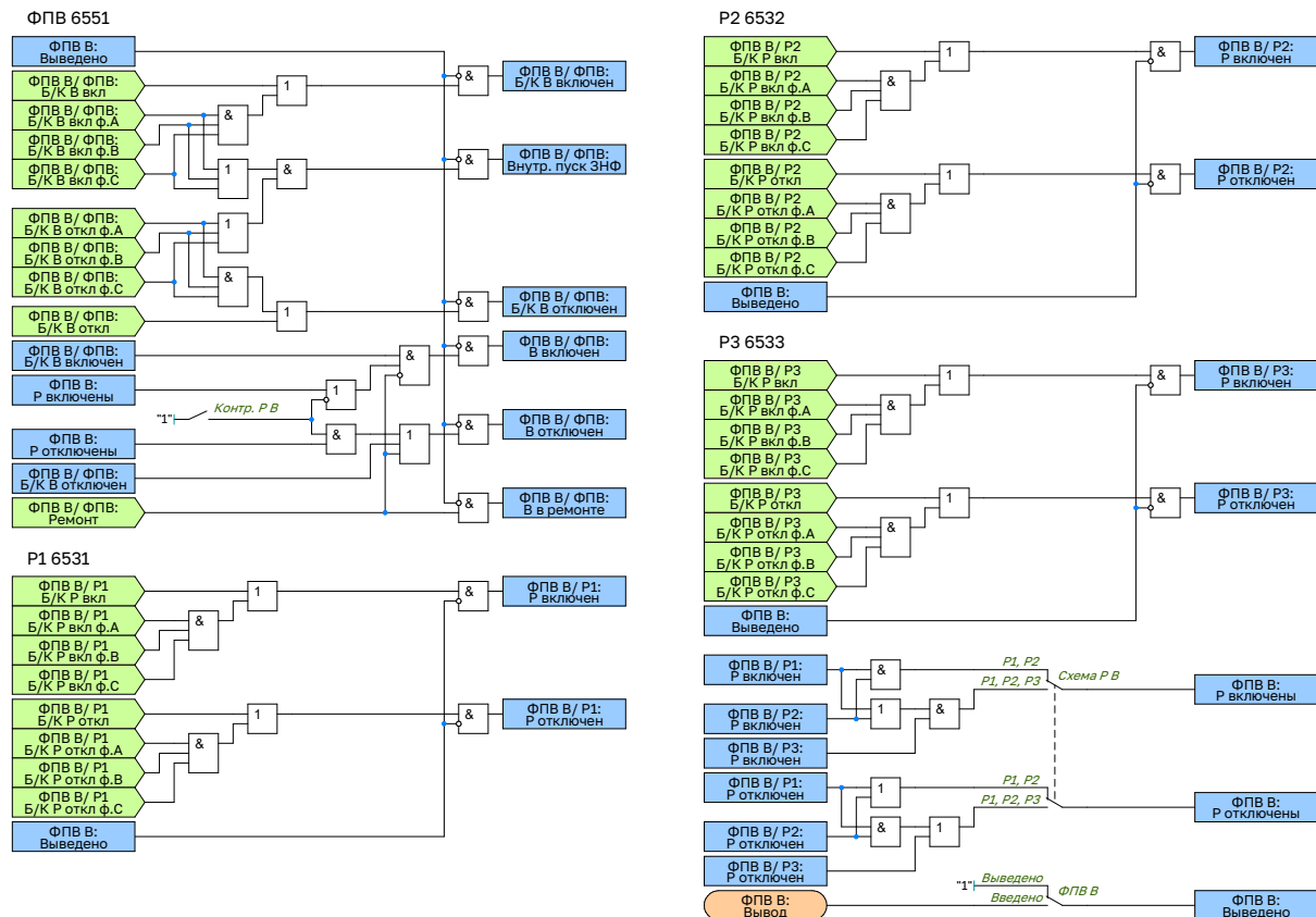
Рисунок 2.60 – Функциональная схема логики ФПВ В1
